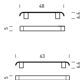
11. K041----, K042---- ДЕРЖАТЕЛЬ ПОЛОТЕНЕЦ, длина 630 или 480 мм, корпус из хромированной латуни.
