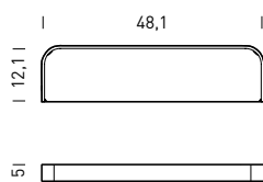
10. K040---- ПОЛКА ДЛЯ ПРЕДМЕТОВ, ширина 480 мм, глубина 120 мм, отделка: хромированная латунь и сталь.
