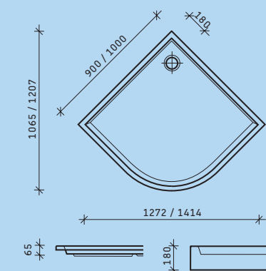
# 720030xx 900 x 900 mm # 720032xx 1000 x 1000 mm
