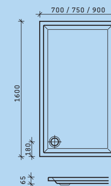
# 720038xx 700 x 1600 mm # 720039xx 750 x 1600 mm # 720040xx 900 x 1600 mm
