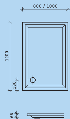
# 720016xx 800 x 1200 mm # 720018xx 1000 x 1200 mm
