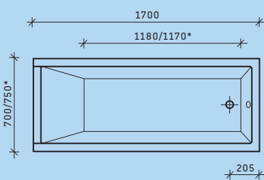
# 700002xx 1700 x 700 mm # 700003xx 1700 x 750 mm*
