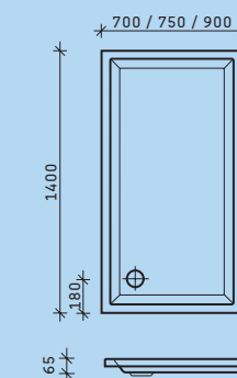
# 720034xx 700 x 1400 mm # 720019xx 750 x 1400 mm # 720035xx 900 x 1400 mm
