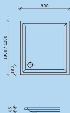
# 720015xx 900 x 1000 mm # 720017xx 900 x 1200 mm
