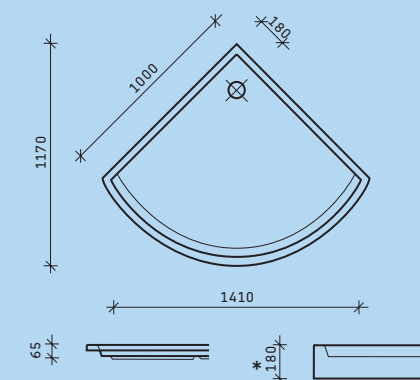
# 720003xx 1000 x 1000 mm # 720004xx 1000 x 1000 mm*
